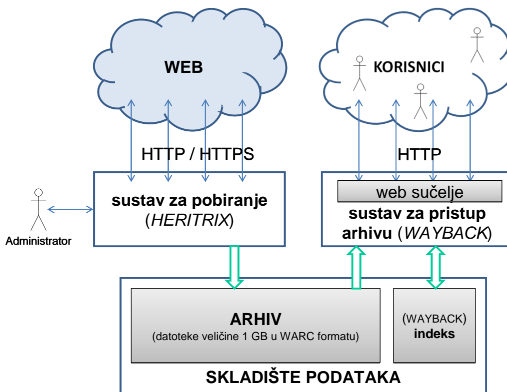
Slika 4. Arhitektura sustava za harvestiranje
