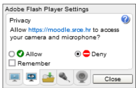
Slika 44. Uključivanje mikrofona
