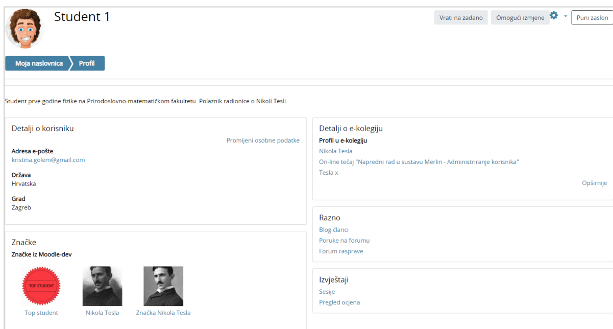
Slika 10. Osobni profil
