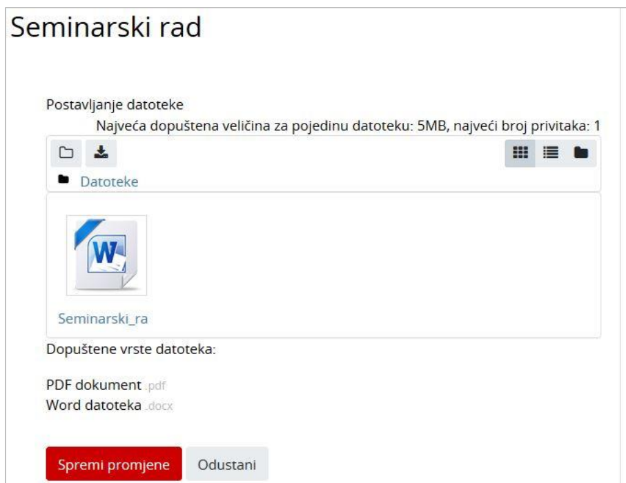
Slika 34. Postavljanje datoteke
